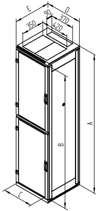
RMA 800 x 800 mm 2 Boxen
